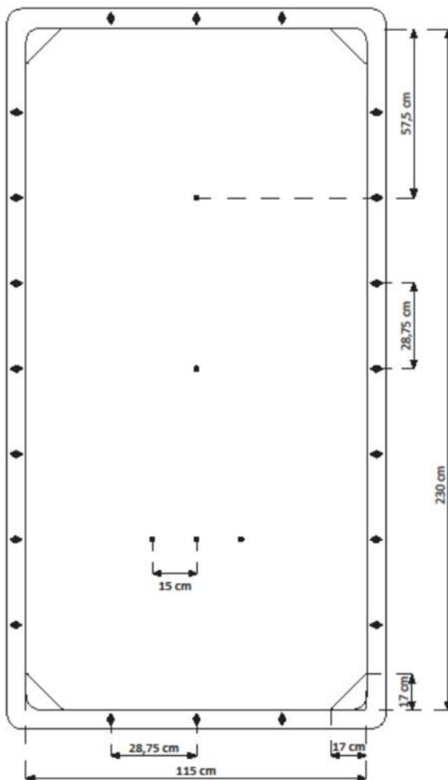
Tekening 2: Verboden zones libre-klein (tot overgangsklasse) en afmetingen klein-biljart
