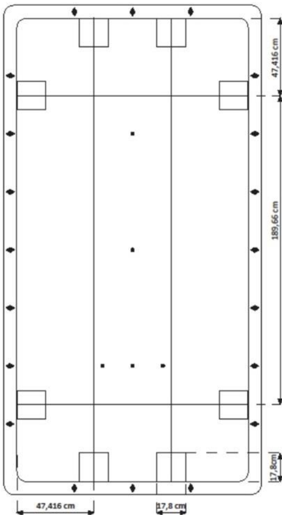
Tekening 8: Afmetingen ankerkader 47/2 groot-biljart
