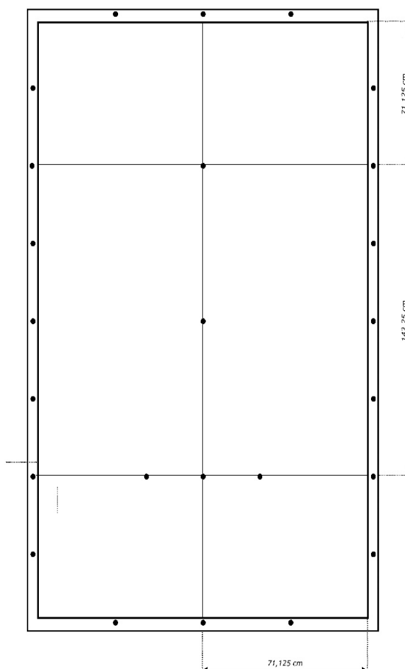
Afmetingen kader 57/2 (tekening 7)
