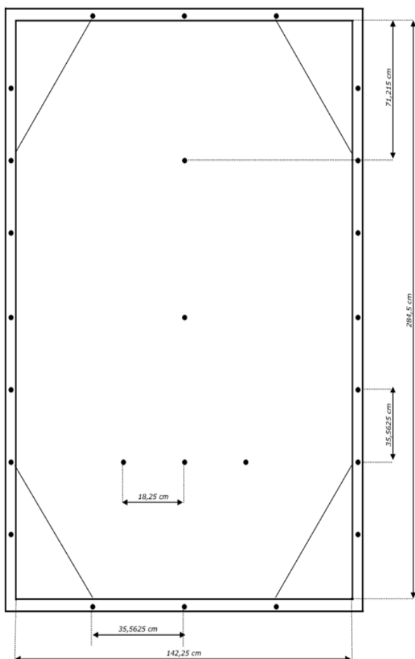
Tekening 5 . Maten grote-tafel met grote hoeken
