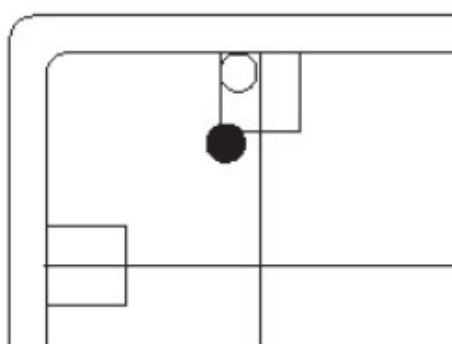
Figuur 4 ankerkader 47/1: dedans-à cheval tweestoots kaderspelsoorten: entree-à cheval* of dedans-à cheval*
