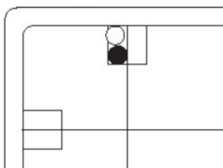
Figuur 3 ankerkader 47/1: dedans-partout tweestoots kaderspelsoorten: entree-dedans* of dedans-entrée* of entree-partout* of dedans-partout*
